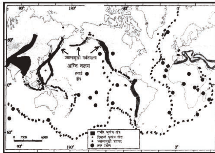
भूकम्प व ज्वालामुखियों का वितरण
