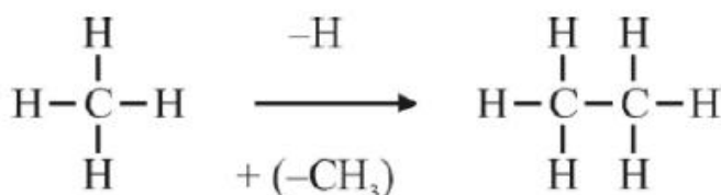
चित्र क्रमांक-2 : एथेन की संरचना
