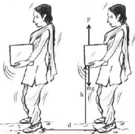
चित्र क्रमांक-8 : विद्यार्थी द्वारा समान उठाते हुए
