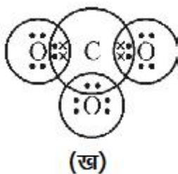
चित्र क्रमांक-1 : (ख) तथा (ग)
