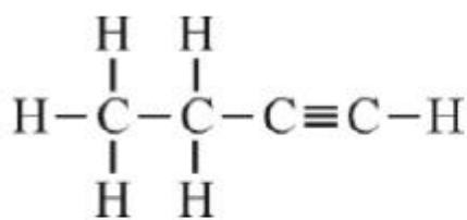
(क) ब्यूट-1-आइन
