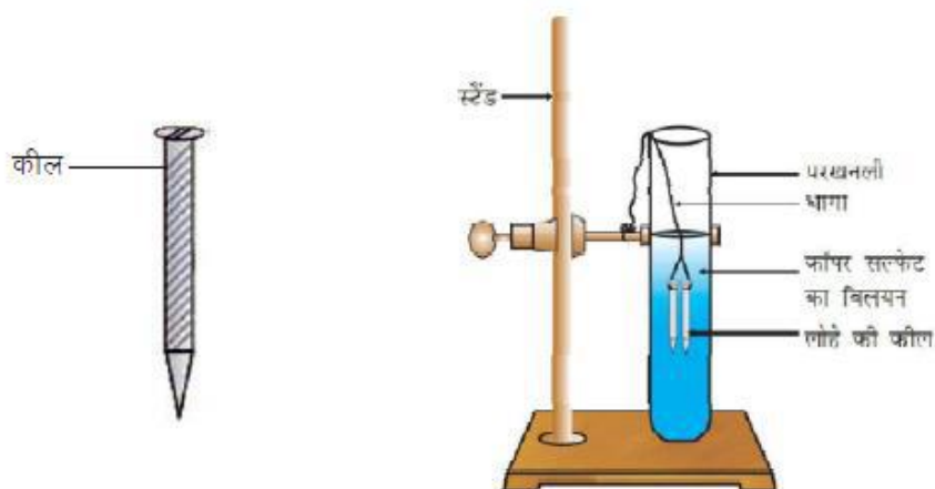
चित्र क्रमांक-5 (अ) : कॉपर सल्फेट के विलयन में डूबी तथा बाहर रखी हुई लोहे की कीलें
