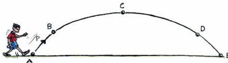
चित्र क्रमांक-3: गेंद च की गति का पथ
