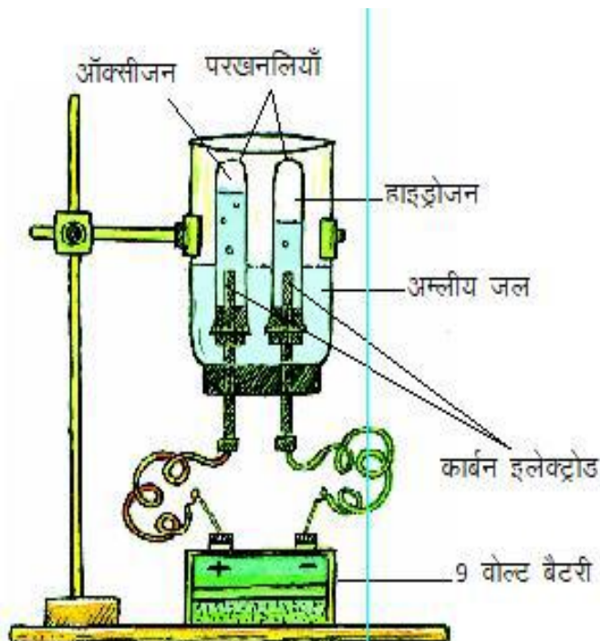
चित्र क्रमांक-7 : जल का विद्युत अपघटन
