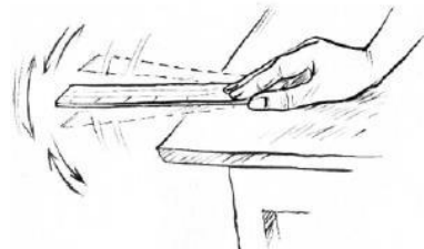
चित्र क्रमांक-1 : मीटर स्केल में कंपन
