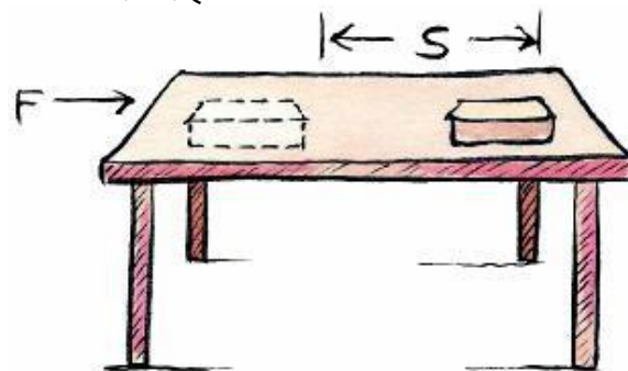
चित्र क्रमांक-10: गति करती हुए वस्तु
