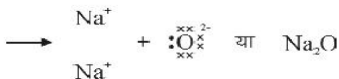
चित्र क्रमांक-5: सोडियम ऑक्साइड का बनना
