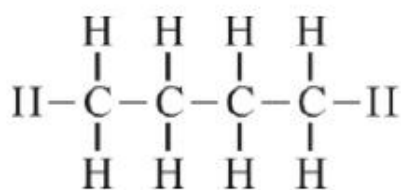
चित्र क्रमांक-5 : (ब्यूटेन)
