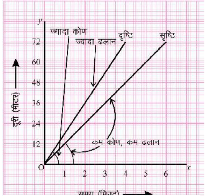
ग्राफ चित्र क्रमांक-5: दृष्टि और सृष्टि का गति का ग्राफ
