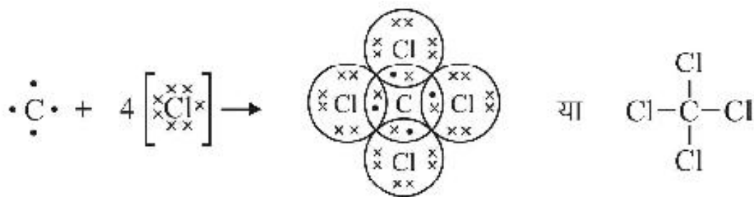
चित्र क्रमांक-6: कार्बन टेट्राक्लोराइड में सहसंयोजकता बंध
