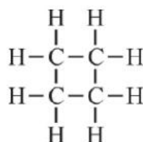
साइक्लोब्यूटेन
