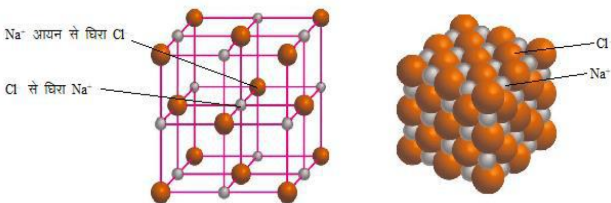
चित्र क्रमांक-1: (ख) सोडियम क्लोराइड की त्रिविमीय संरचना
