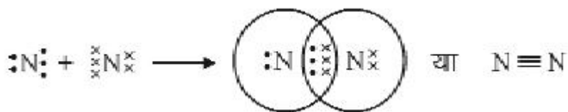
चित्र क्रमांक-14: नाइट्रोजन में सहसंयोजक बंध
