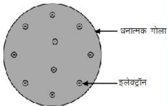
चित्र क्रमांक-4 थॉमसन का परमाणु मॉडल
