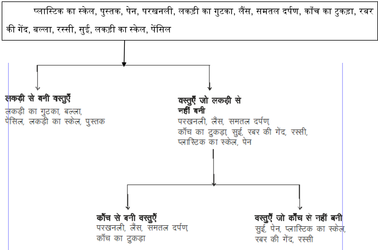
चित्र क्रमांक-1: वस्तुओं का वर्गीकरण
