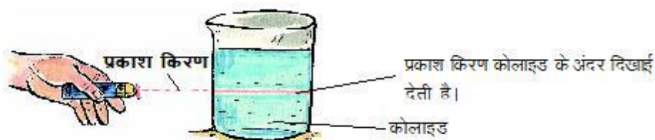
चित्र क्रमांक-5 : टिंडल प्रभाव
