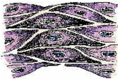
अरेखित पेशीय ऊतक (unstriated muscle tissue) (स) पेशीय ऊतक (Muscular tissue)
