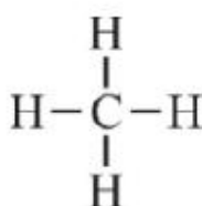
चित्र क्रमांक-1 : मेथेन की संरचना
