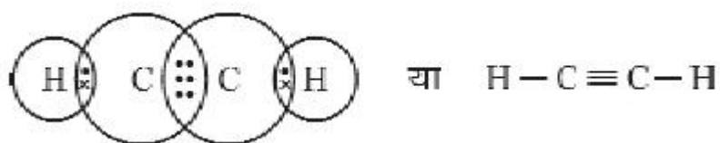
चित्र क्रमांक-15: एथाइन में सहसंयोजक बंध
