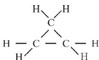
साइक्लोप्रोपेन
