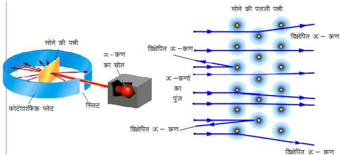
(क) रदरफोर्ड का प्रकीर्णन प्रयोग
