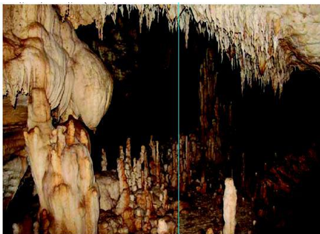
चित्र क्रमांक-1: कुटुमसर गुफा की शंकु जैसी रचनाएँ-छत से लटकते स्टैलेक्टाइट एवं जमीन से उभरते स्टैलेक्माइट
