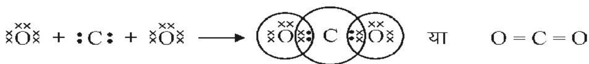
चित्र क्रमांक-8: कार्बन डाइऑक्साइड में सहसंयोजक बंध
