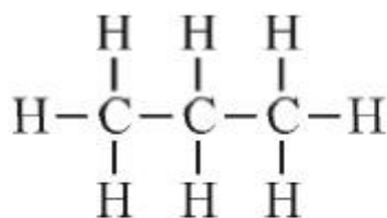
चित्र क्रमांक-3 : तीन कार्बन परमाणु वाली शृंखला
