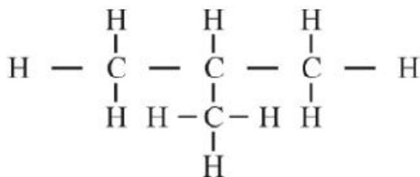
चित्र क्रमांक-6 : (2-मेथिलप्रोपेन)
