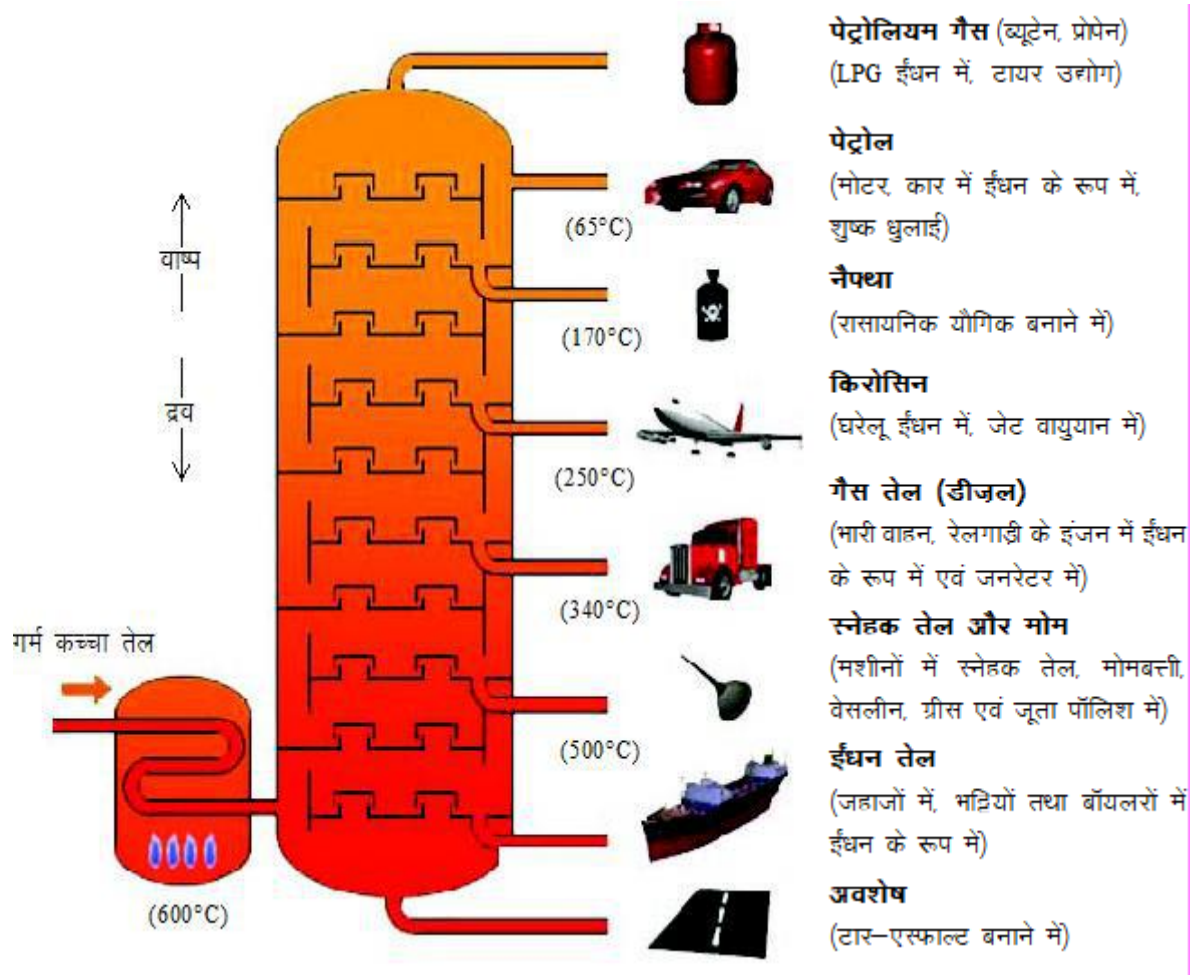
चित्र क्रमांक-3: पेट्रोलियम का प्रभाजी आसवन
