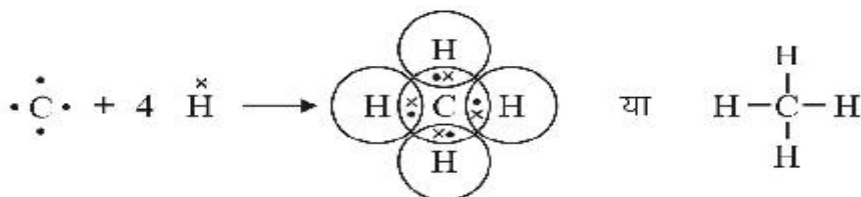
चित्र क्रमांक-7: मेथेन में सहसंयोजक बंध
