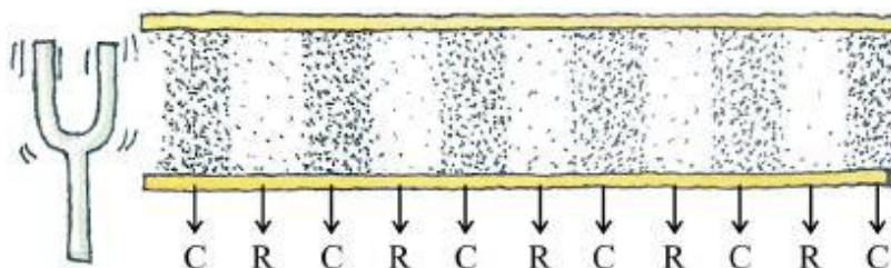
चित्र क्रमांक-4: कंपित स्वरित्र त्रिभुज में क्रमशः संपीड़न तथा विरलन की शृंखला (यहाँ C संपीड़न तथा R विरलन को दर्शाता है।)
