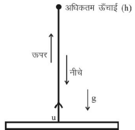
चित्र क्रमांक-4 : गेंद की गति
