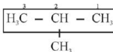
चित्र क्रमांक-8: (2-मेथिलप्रोपेन)
