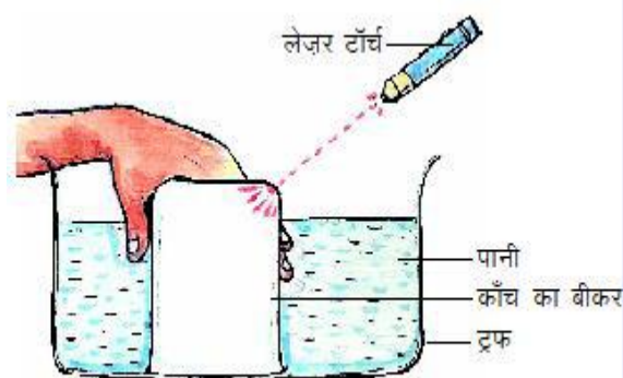
चित्र क्रमांक-1 : पदार्थ स्थान घेरता है
