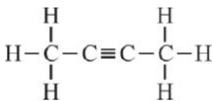
(ख) ब्यूट-2-आइन
