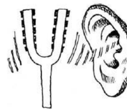
चित्र क्रमांक-3 : कंपित स्वरित्र द्विभुज की ध्वनि सुनना
