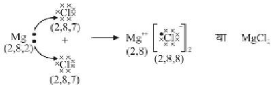
चित्र क्रमांक-2: मैग्नीशियम क्लोराइड का बनना
