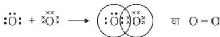
चित्र क्रमांक-12: ऑक्सीजन में सहसंयोजक बंध
