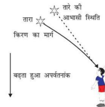
चित्र 11.9 वायुमंडलीय अपवर्तन के कारण तारे की आभासी स्थिति
