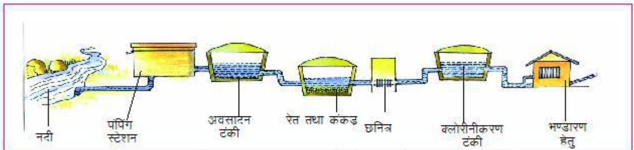
चित्र 4.10 (ब) जल संस्थानों में जल को शुद्ध करने की विधि
