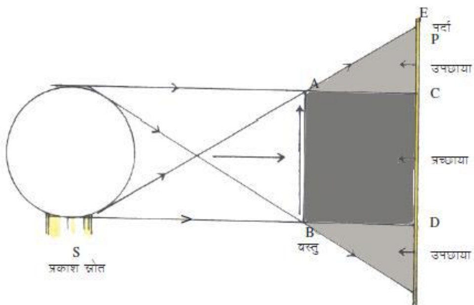
चित्र-12.6 छाया तथा उपछाया का बनना
