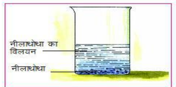
चित्र 4.12 नीलाथोथा का क्रिस्टलीकरण
