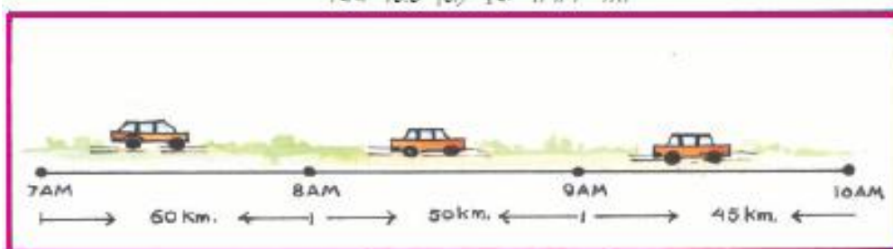
चित्र 10.6 (ब) असमान गति
