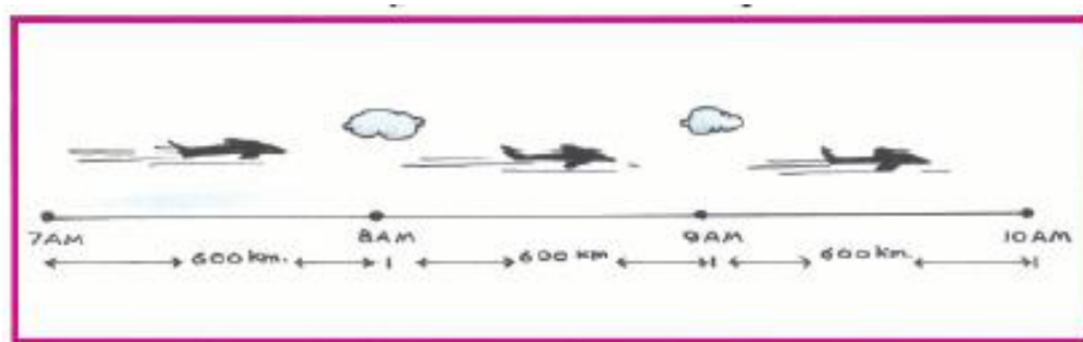
चित्र 10.6 (अ) एक समान गति
