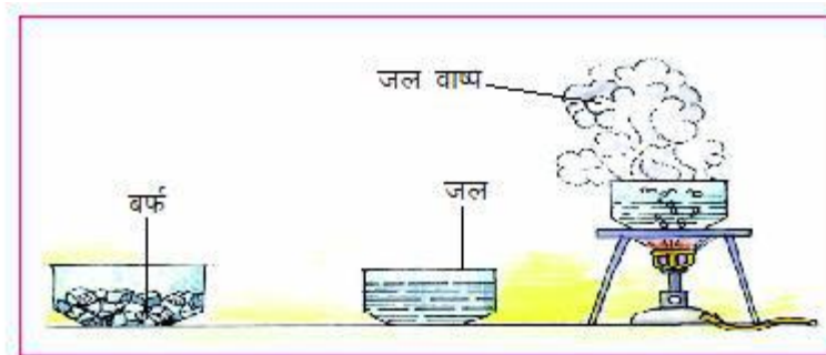
चित्र 5.3 भौतिक परिवर्तन
