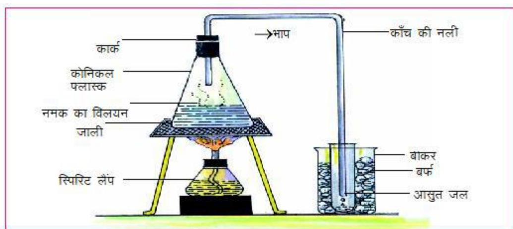
चित्र 4.13 आसवन
