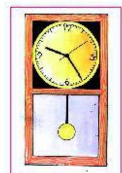
चित्र 5.2 आवर्ती परिवर्तन
