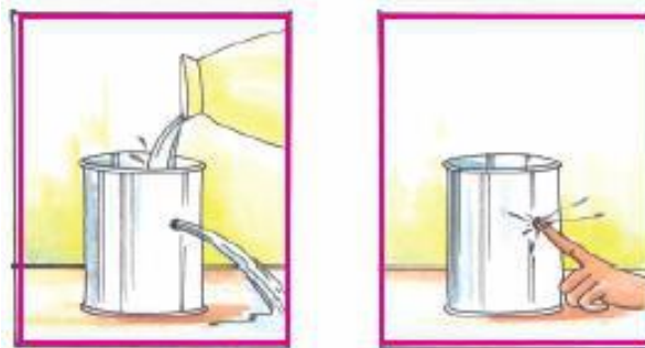
चित्र 10.13 द्रव का दाब
