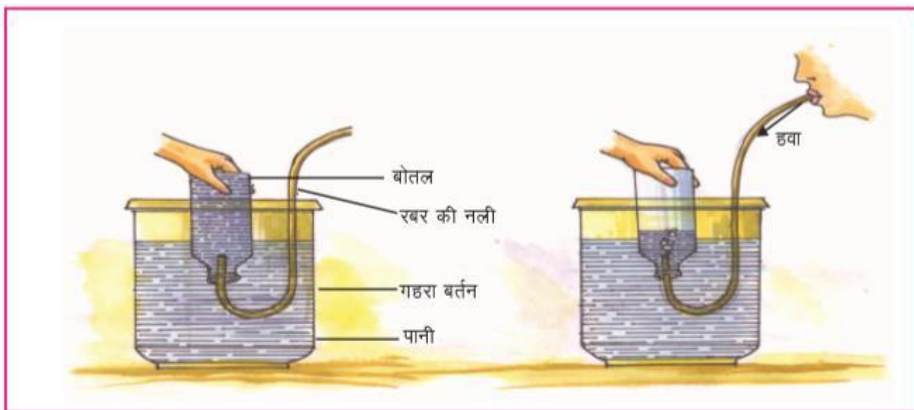
चित्र 3.2 गैसों स्थान घेरती हैं
