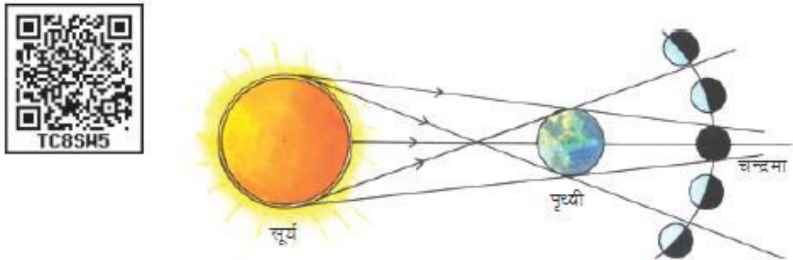
चित्र 12.7 चंद्र ग्रहण
