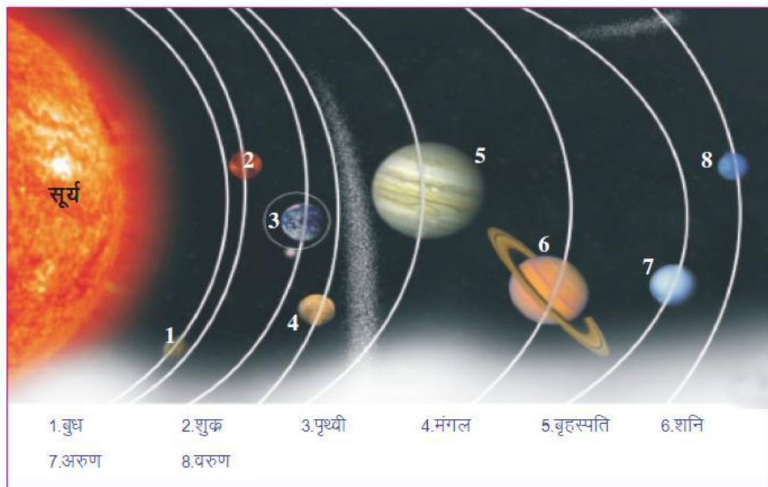
चित्र 1.4 सौर परिवार
