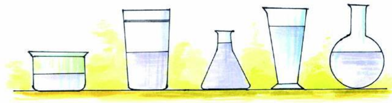
चित्र 3.1 विभिन्न आकार के बर्तन
