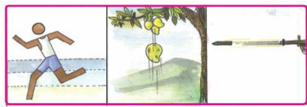
चित्र-10.2 सरल रेखीय गति के उदाहरण
