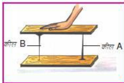
चित्र-10.12 दाब का प्रभाव
