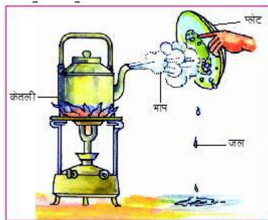
चित्र- 5.1 उत्क्रमणीय परिवर्तन
