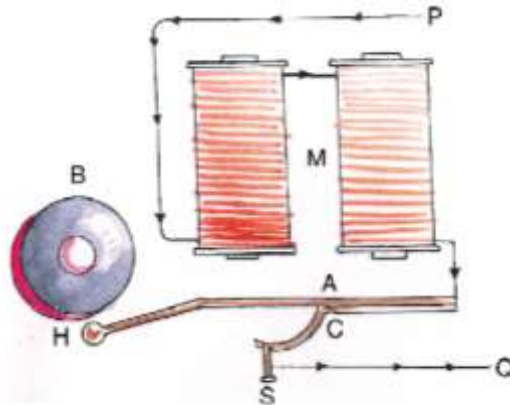
चित्र 21.9 विद्युत घंटी
