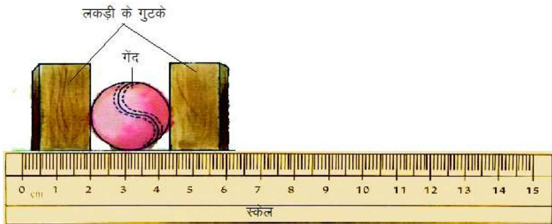
चित्र-5.3 गोलाकार वस्तु का व्यास ज्ञात करना
