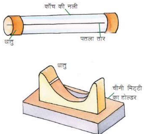
चित्र 21.6 सुरक्षा फ्यूज
