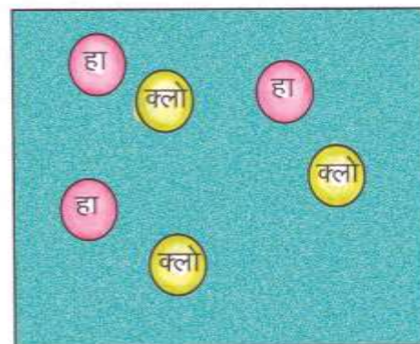
चित्र 5 हाइड्रोजन एवं क्लोरीन के परमाणु
