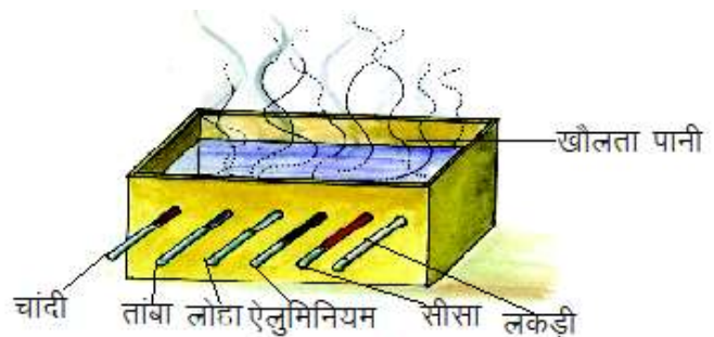
चित्र-8.3 ऊष्मा का सर्वोत्तम चालक
