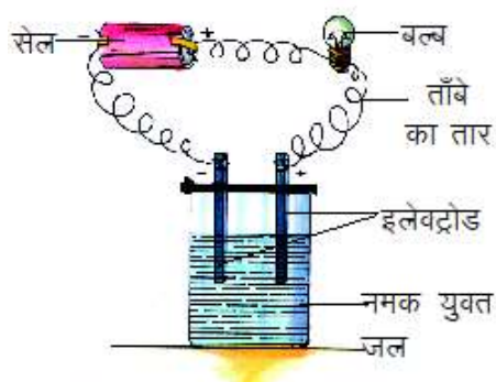
चित्र-2.3 विद्युत चालकता
