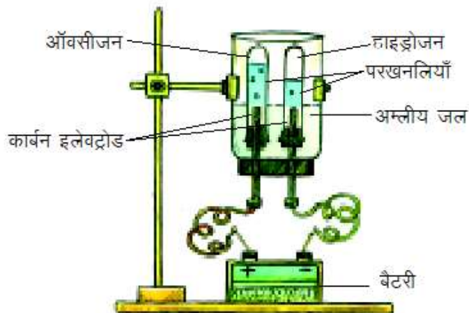
चित्र-2.4 जल का विद्युत अपघटन
