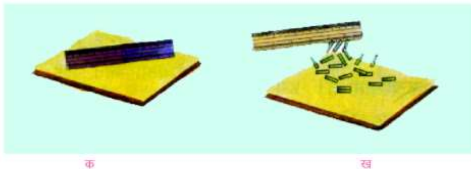
चित्र-15.3 सम्पर्क द्वारा आवेशन
