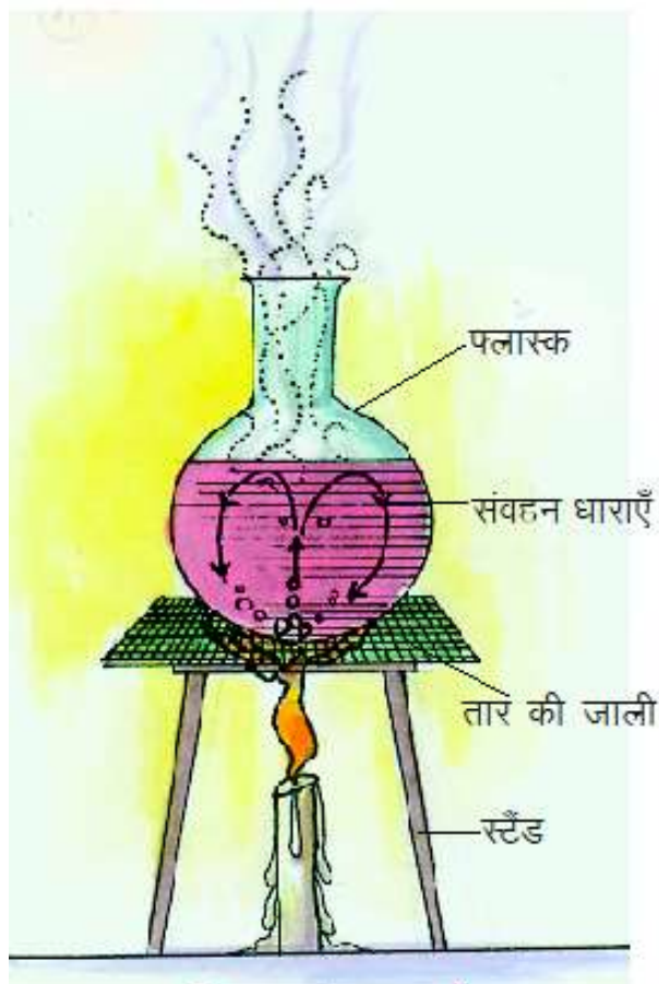
चित्र-8.4 संवहन धाराएँ
