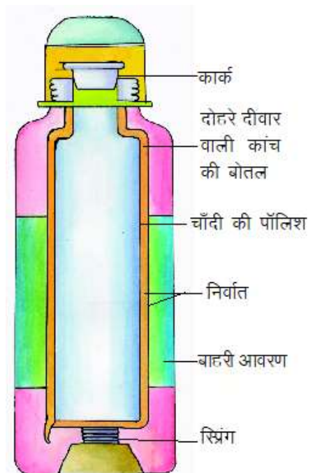
चित्र-8.9 थर्मस फ्लास्क
