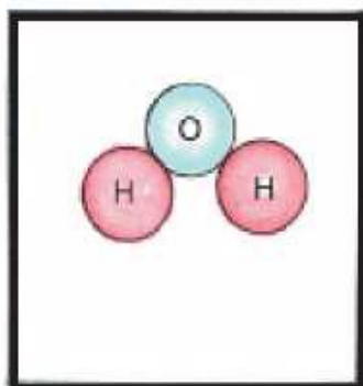
चित्र 3.9 क पानी का एक अणु
