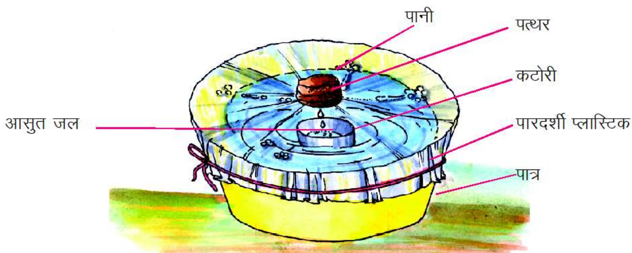
चित्र-2.2 आसुत जल एकत्र करना
