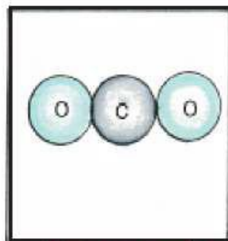
चित्र 3.9 ख कार्बन डाइऑक्साइड का एक अणु
