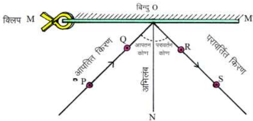
चित्र-12.4 परावर्तन के नियम का सत्यापन
