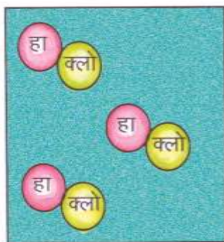
चित्र 4 हाइड्रोक्लोरिक अम्ल के अणु
