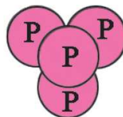
चित्र 3.8 फास्फोरस का एक अणु
