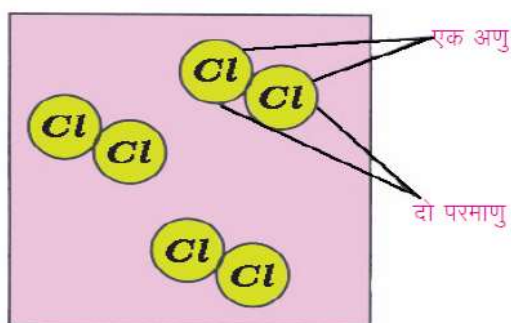
चित्र 3.7 क्लोरीन के तीन अणु
