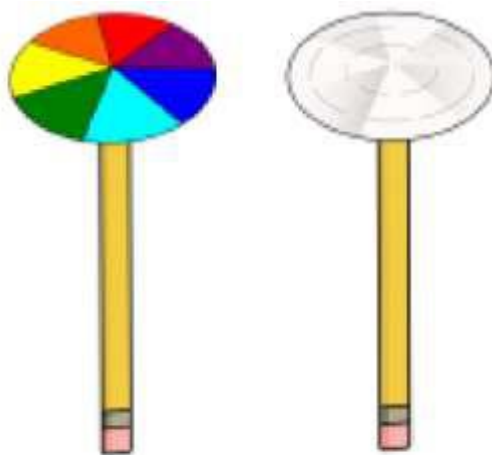
चित्र 12.22 (क) सात वर्णों वाली डिस्क
