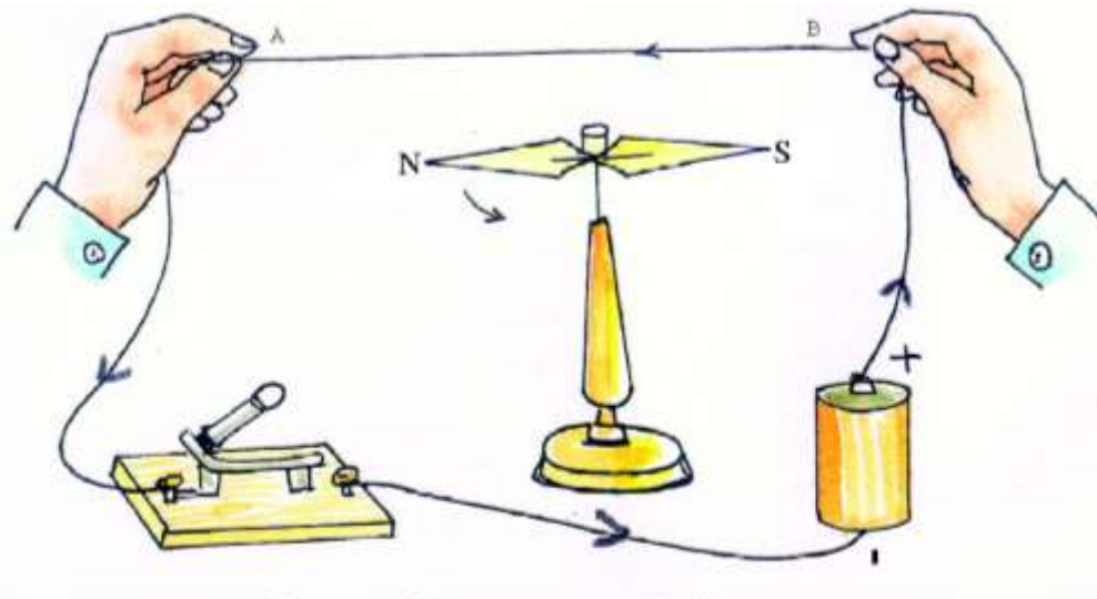
चित्र 21.7 विद्युत धारा का चुंबकीय प्रभाव।
