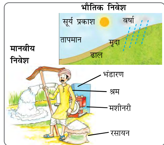
चित्र 4.3 : भौतिक एवं मानवीय कृषि निवेश
