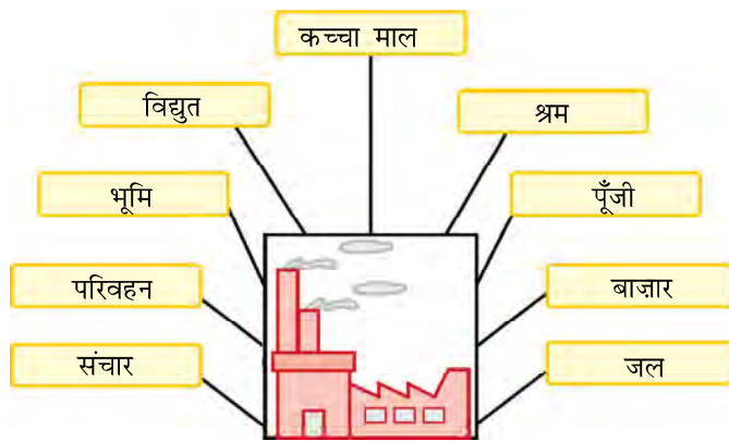
चित्र 5.3 : उद्योगों के अवस्थिति संबंधी कारक
