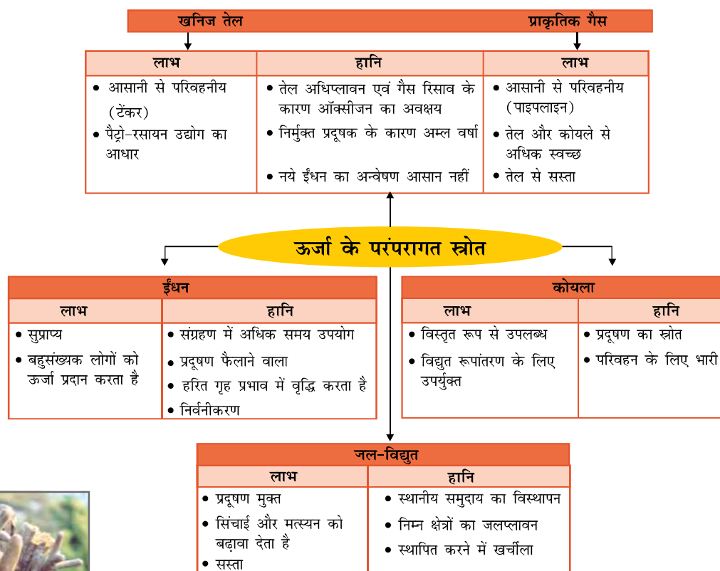
चित्र 3.8: ऊर्जा के परंपरागत स्रोत
