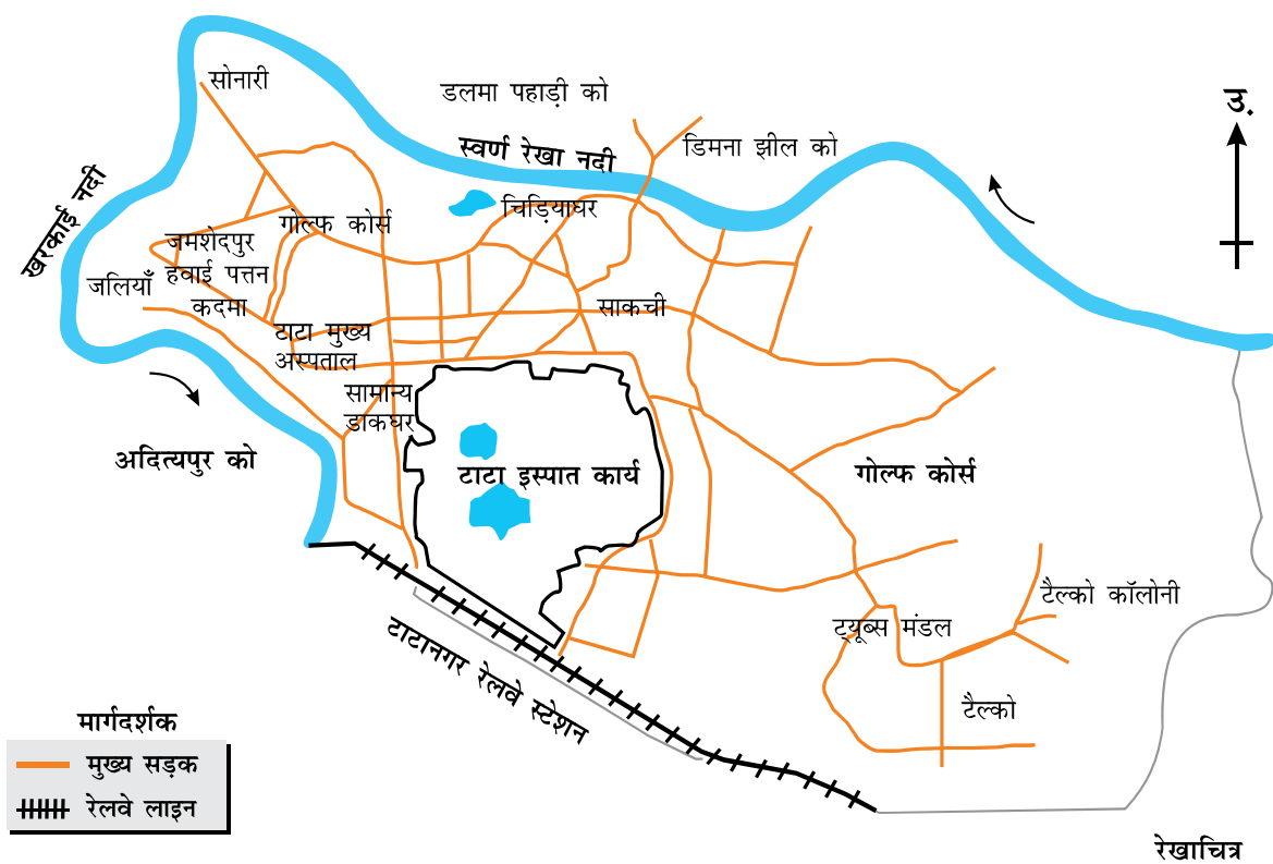
चित्र 5.9 : जमशेदपुर में लोहा-इस्पात उद्योग की अवस्थिति
