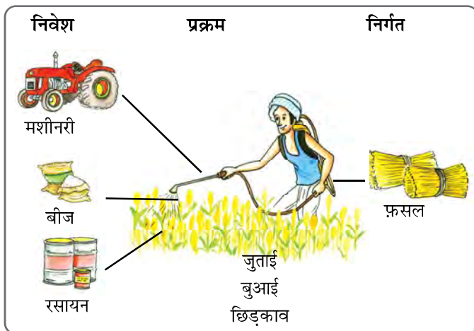
चित्र 4.2 : कृषिगत भूमि की कृषि पद्धति
