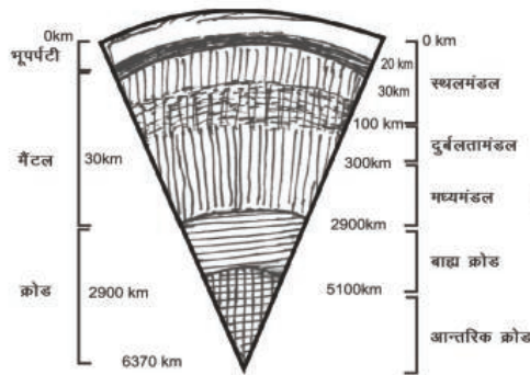
चित्र : पृथ्वी की आंतरिक संरचना
