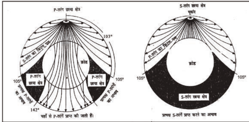
चित्र : भूकम्पीय छाया क्षेत्र
